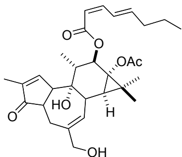
Pedilstatin
