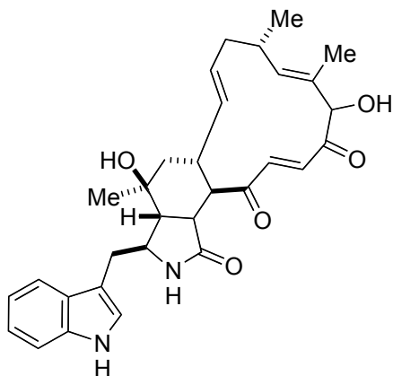
Chaetoglobosin Q
