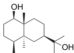
(±)-balanitol
